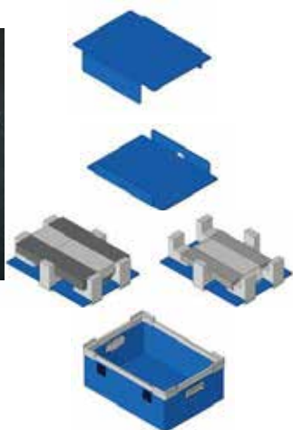
【中型製品サイズ規格ボックス】 ・可変式パッド構造で 幅広い製品サイズに対応可能 ・返却時は折りたたみ可能
